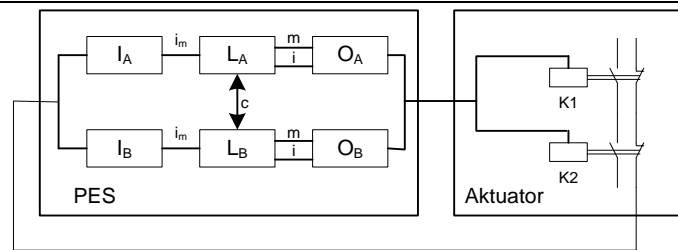
Einkanaliger Ausgang SMX mit intern zweikanaliger Verarbeitung (IQQx) und zweikanaliger Aktuator mit zweikanaliger Diagnose
