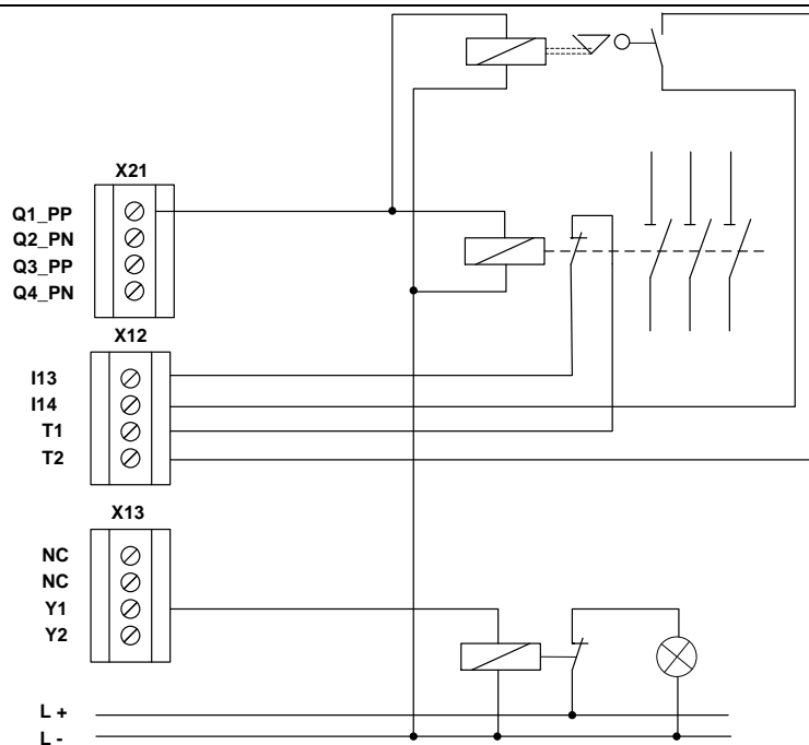
Bild: Einkanalig schaltender Ausgang Q1_PP mit zweikanaligem externem Kreis als Kombination elektromechanisches Element und hydraulisches/pneumatisches Ventil und Überwachung an zwei Eingängen
