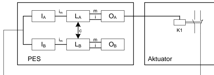
Einkanaliger Ausgang SMX und einkanaliger Aktuator mit Diagnose
