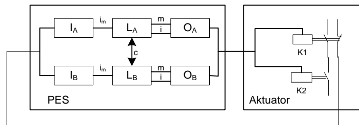
Einkanaliger Ausgang SMX mit intern zweikanaliger Verarbeitung (IQQx) und zweikanaliger Aktuator mit mind. einkanaliger Diagnose
