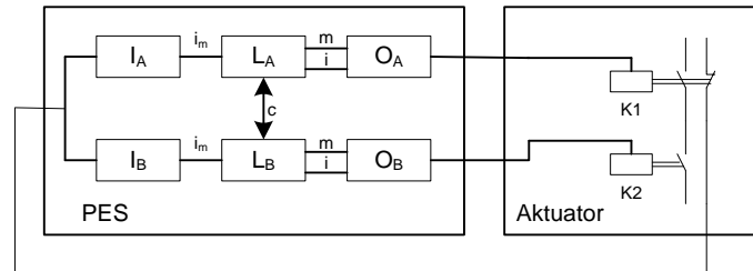
Zweikanaliger Ausgang SMX und zweikanaliger Aktuator mit einkanaliger Diagnose
