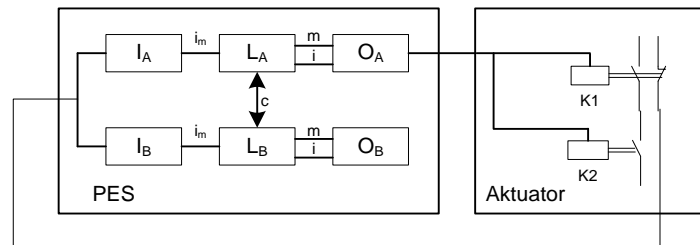
Einkanaliger Ausgang SMX (Rel 1 / 2, DO 0/1P, DO 0/1M) und zweikanaliger Aktuator mit mind. einkanaliger Diagnose
