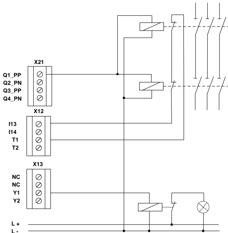
Bild: Einkanalig schaltender Ausgang Q1_PP mit zweikanaligem externem Kreis und Überwachung an Eingang 13 als Sammelrückmeldung
