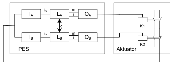
Zweikanaliger Ausgang SMX und zweikanaliger Aktuator mit zweikanaliger Diagnose
