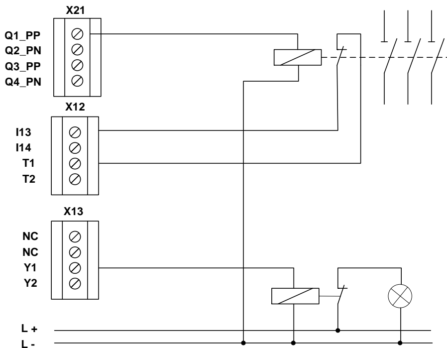
Bild: Einkanalig schaltender Relaisausgang mit Testung
