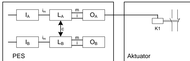
Einkanaliger Ausgang SMX und einkanaliger Aktuator ohne Diagnose
