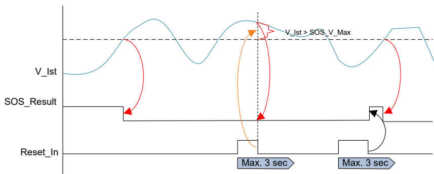
Abbildung 42: Reset-Funktion 2
