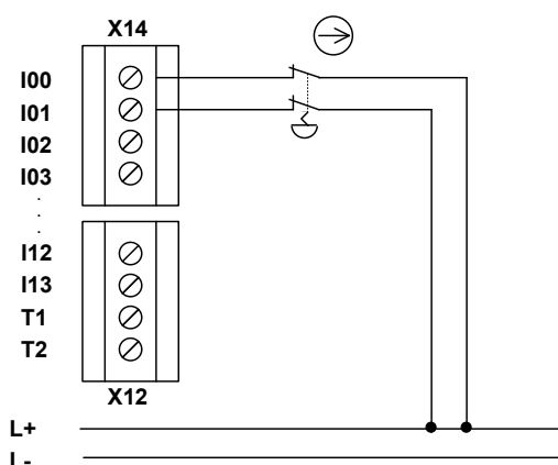
Abbildung 18 zweikanaliger Sensor homogen ohne Taktung, mit Zwangstrennung
