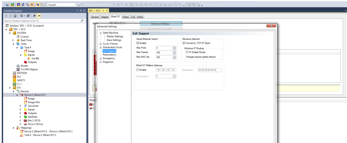
Abbildung 57: TwinCAT - EoE-Einstellung
