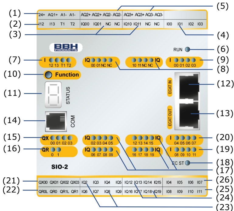
Abbildung 8: Aufbau SIO-2
