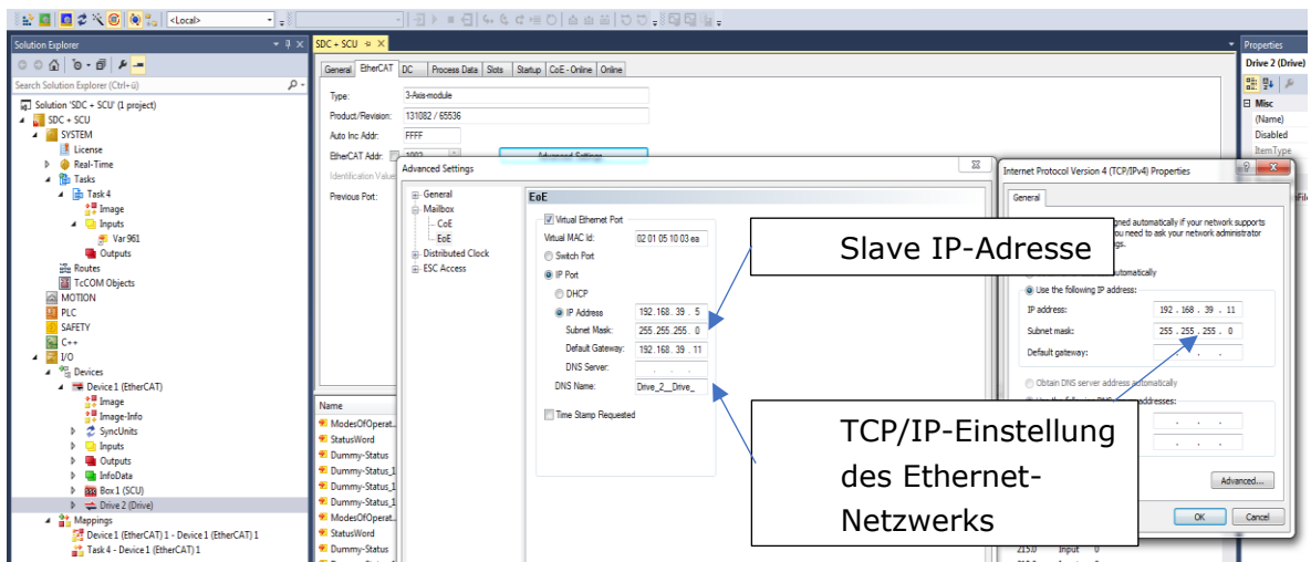
Abbildung 58: TwinCAT - IP-Ports
