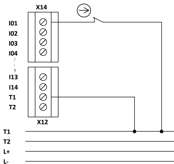
Abbildung 17 Einkanaliger Sensor mit Taktung
