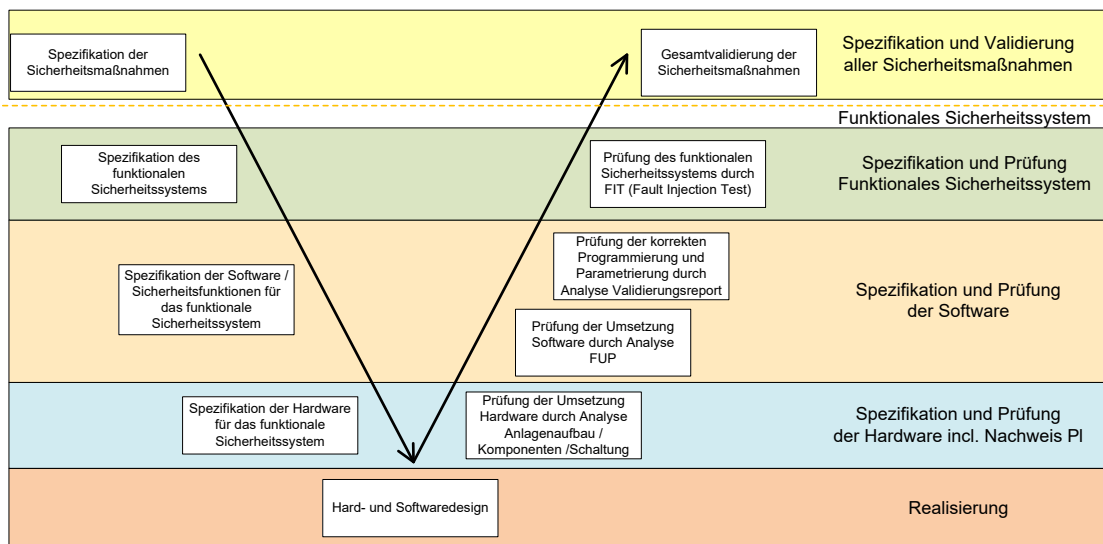
Abbildung 64 V-Modell
