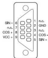
SIN/COS
