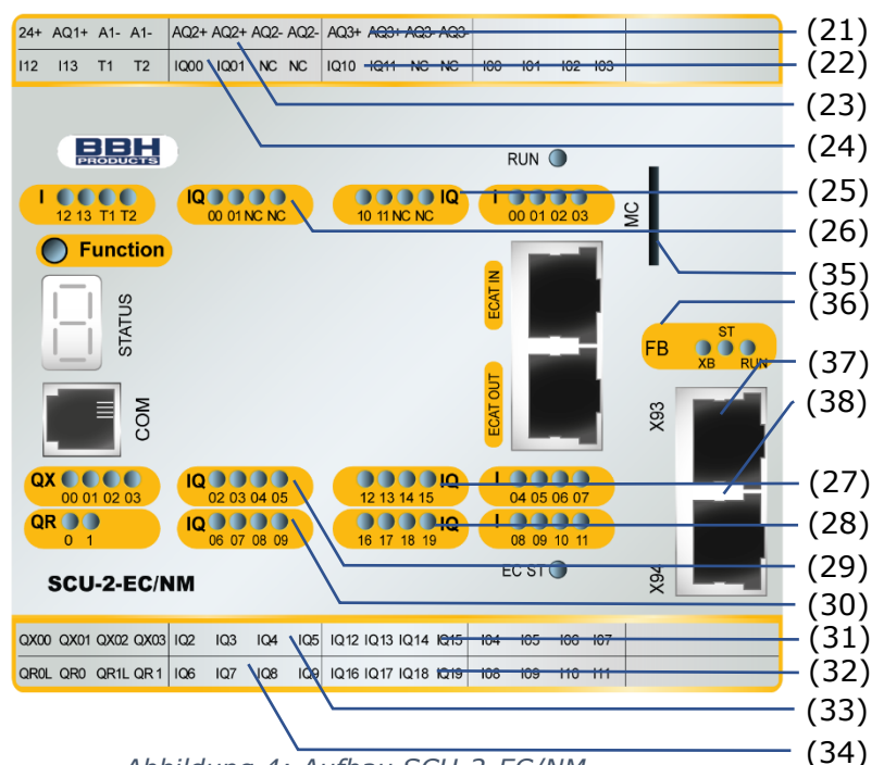
Abbildung 4: Aufbau SCU-2-EC/NM
