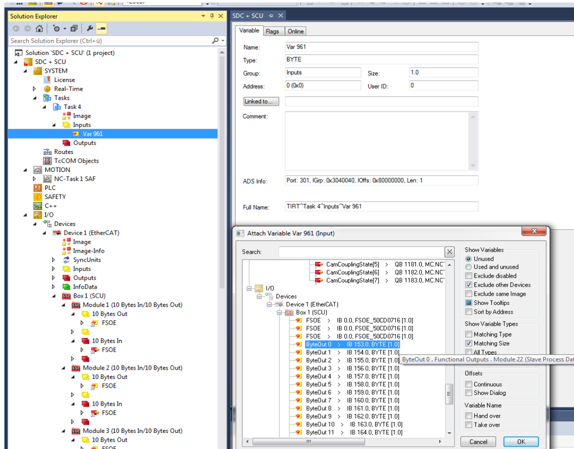
Abbildung 54: TwinCAT - Verbindung
