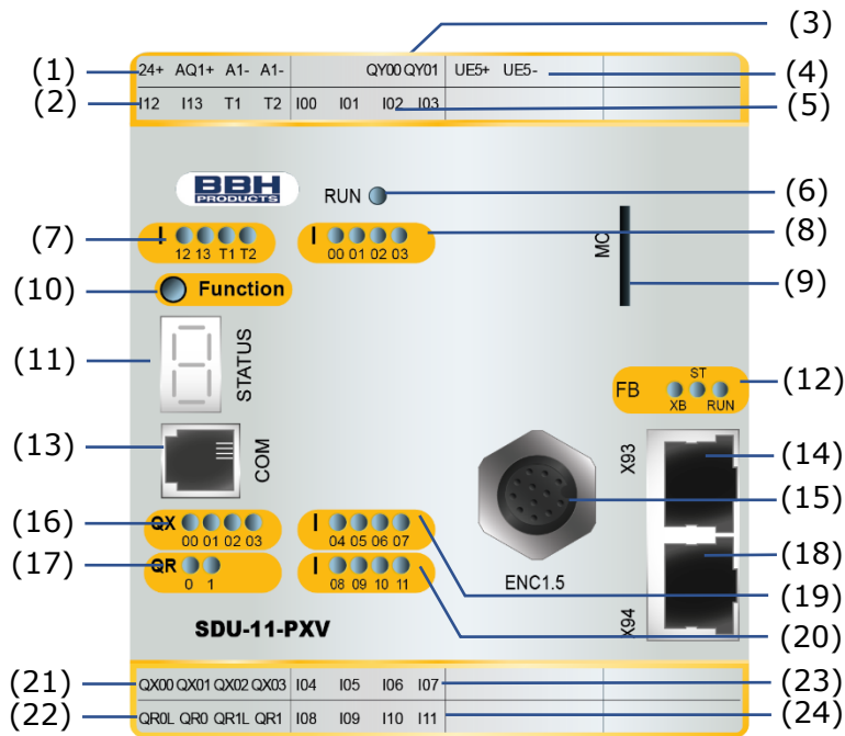
Abbildung 6: Aufbau SDU-11-PXV
